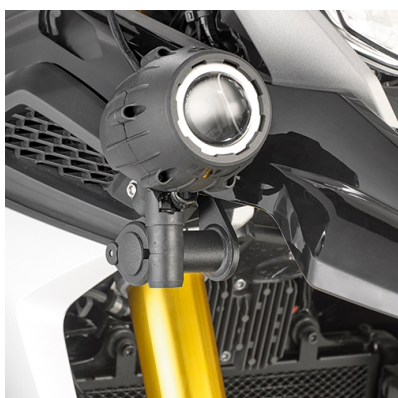
LS5126K Kit d'attaches spécifiques pour les projecteurs halogènes où les pare-carters tubulaires spécifiques ne sont pas présents
