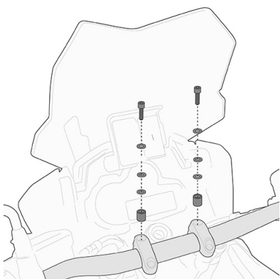
05SKITK Kit de fixation spécifique pour Smart Bar KS900A
