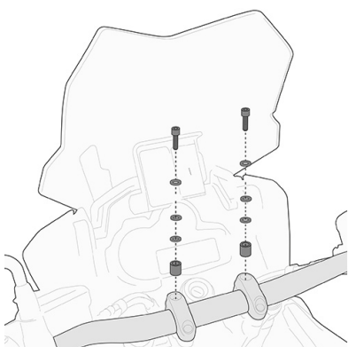
01SKITK Kit viteria specifico per montare lo Smart Bar KS900A
